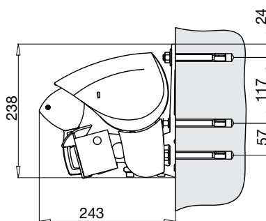
Väggmontage
